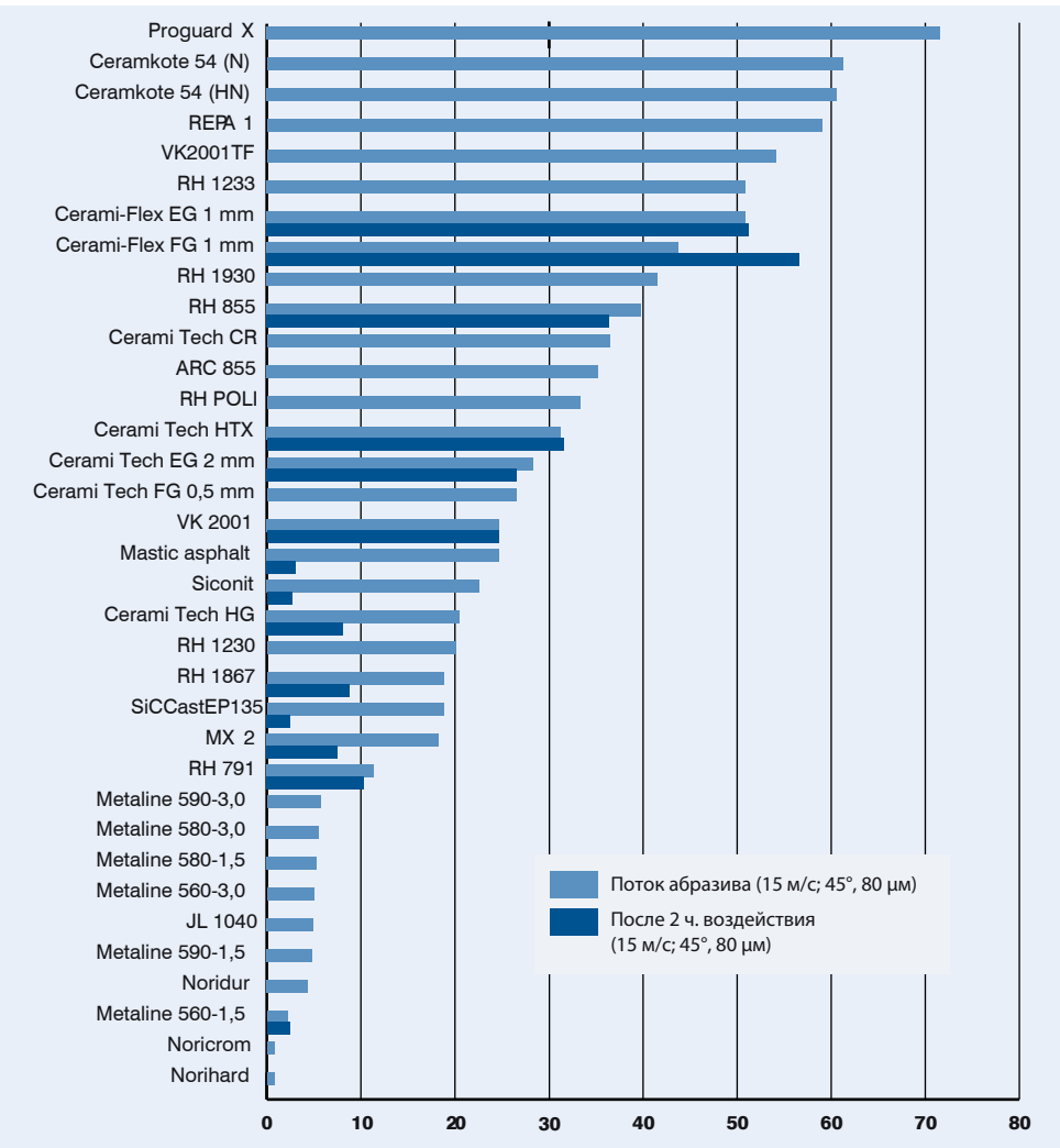
Диаграмма 1: результаты износа покрытий
