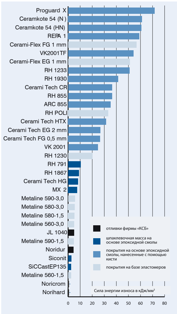
Диаграмма 2: результаты износа покрытий (15 м/с; 45°, 80 μm) (в статическом состоянии под потоком после 2 ч воздействия)
